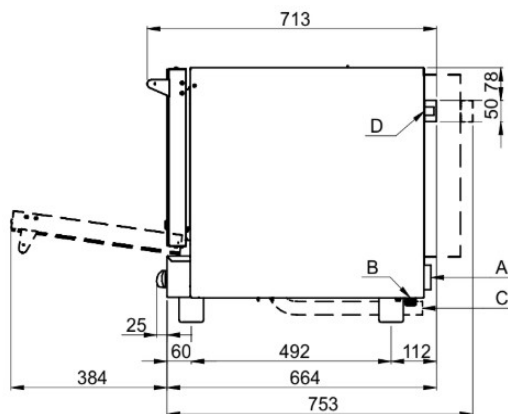
Vue côté porte ouverte
